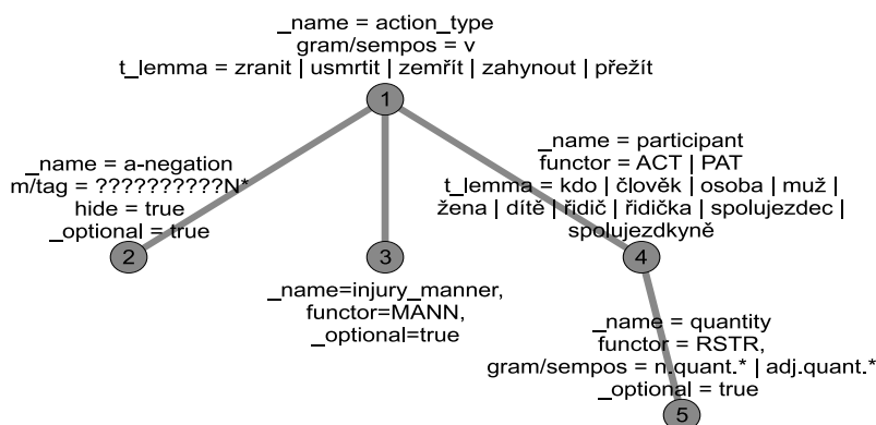
Obr. 2. Netgraph dotaz – extrakční pravidlo.
